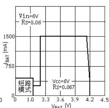
充电电流与电池电压关系
