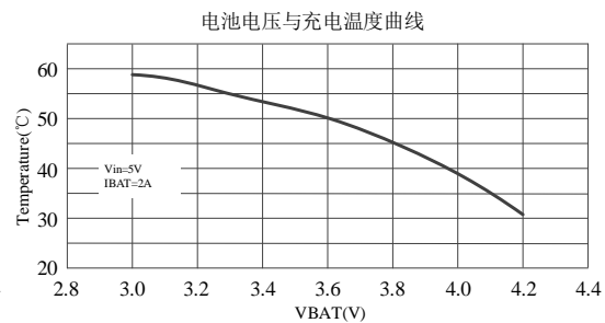
电池电压与充电温度曲线
