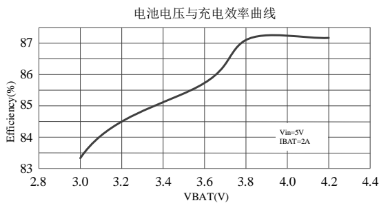
电池电压与充电效率曲线
